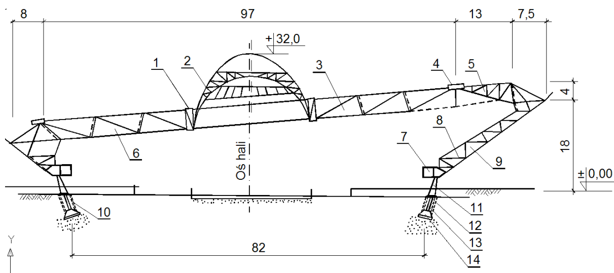
Rysunek 2: Schematyczny przekrój poprzeczny przez konstrukcję przekrycia dachowego: 1 – stalowy pierścień wewnętrzny, 2 – kopuła, 3 – kondygnacja techniczna, 4 – stalowy pierścień zewnętrzny, 5 – wsporniki kratowych żeber obudowy, 6 – dźwigar linowo-prętowy, 7 – żelbetowy, sprężony pierścień fundamentowy, 8 – żelbetowe pierścienie obudowy, 9 – żebra stalowe, 10 – obudowa wahaczy, 11 – słupy krzyżakowe, 12 – pierścień pośredni, 13 – słupy wahaczowe, 14 – stopy fundamentowe
