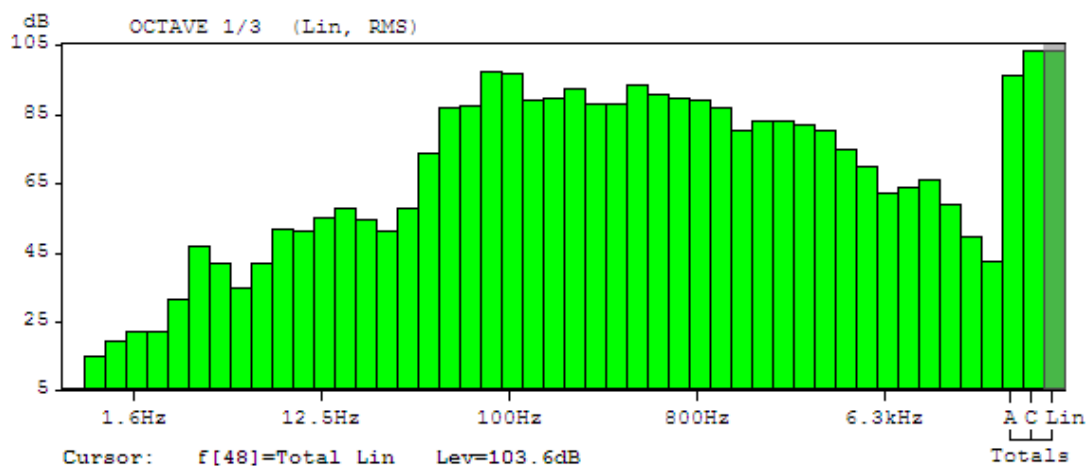
Rysunek 5: Wartości poziomu ciśnienia akustycznego w funkcji częstotliwości dla nagłośnienia typu „głośna muzyka”
