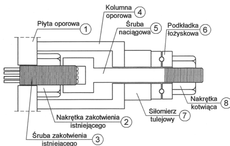
Rysunek 5: Przekrój elementów kotwiących kabel sprężający (9 drutów \phi 5\text{mm} ) z zamontowanym siłomierzem
