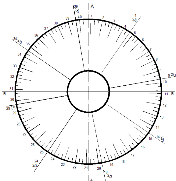
Rysunek 4: Schemat rozmieszczenia dźwigarów ze wskazaniem dźwigarów, w których prowadzone mogą być pomiary kontrolne
