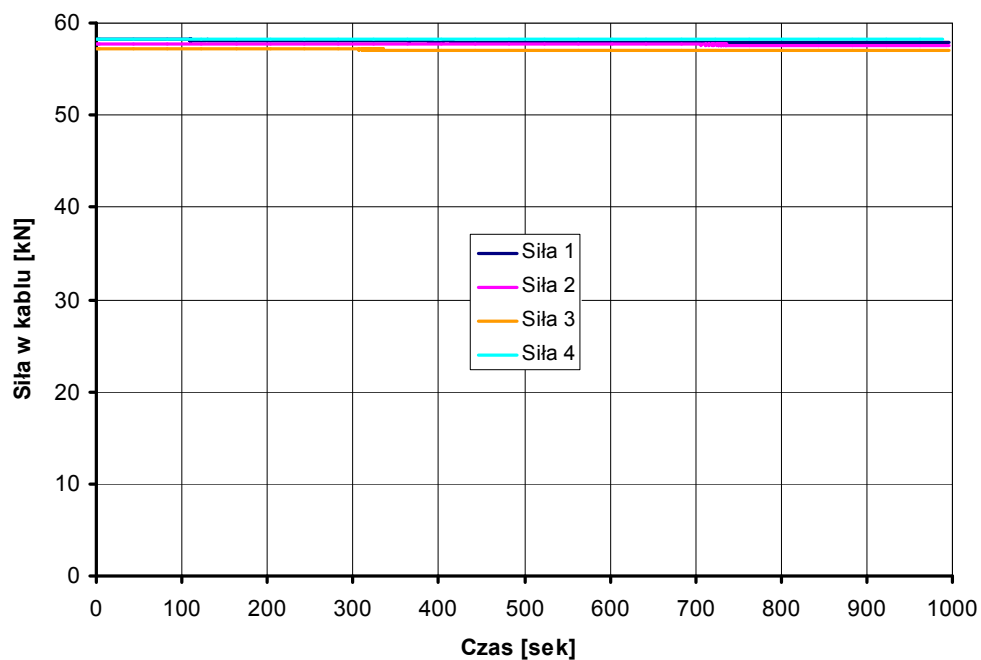
Rysunek 7: Zmiany wartości sił w kablach zarejestrowane podczas trwania oddziaływania fali akustycznej
